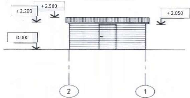
ФАСАД 2-1
