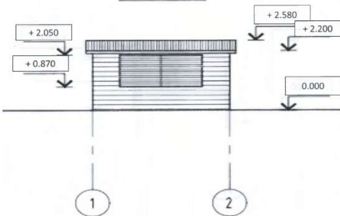
ФАСАД 1-2
