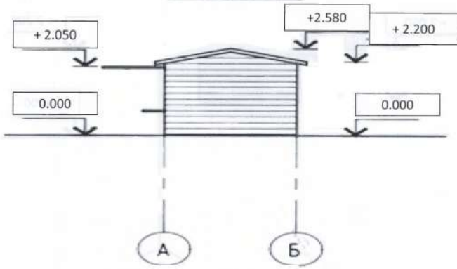
ФАСАД А-Б
