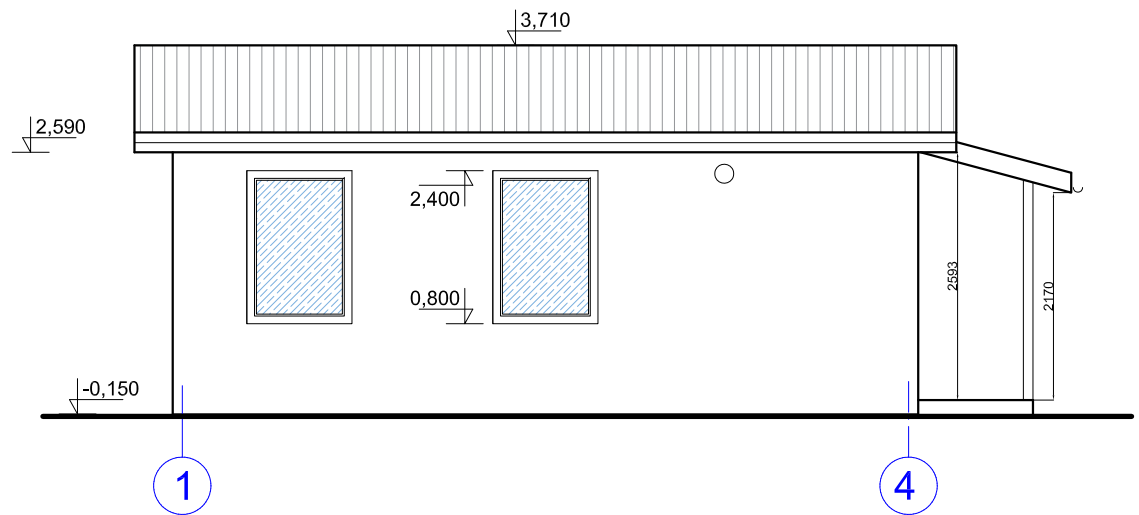
ФАСАД 1 - 4
