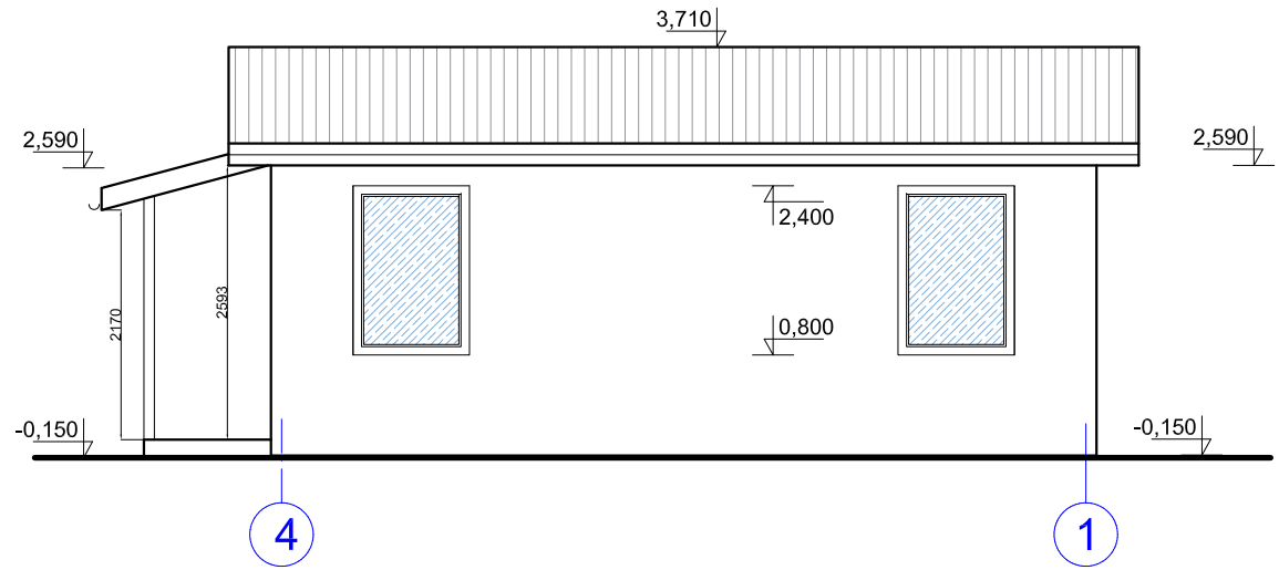
ФАСАД 4 - 1
